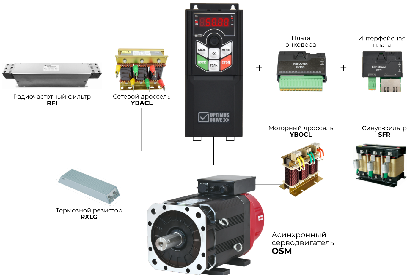
Преобразователь частоты AD800
