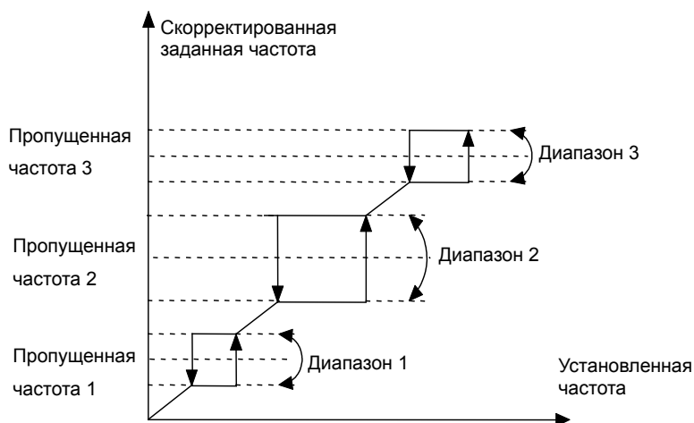
Рис. 6-7 Пропущенные частоты и диапазоны пропущенных частот
