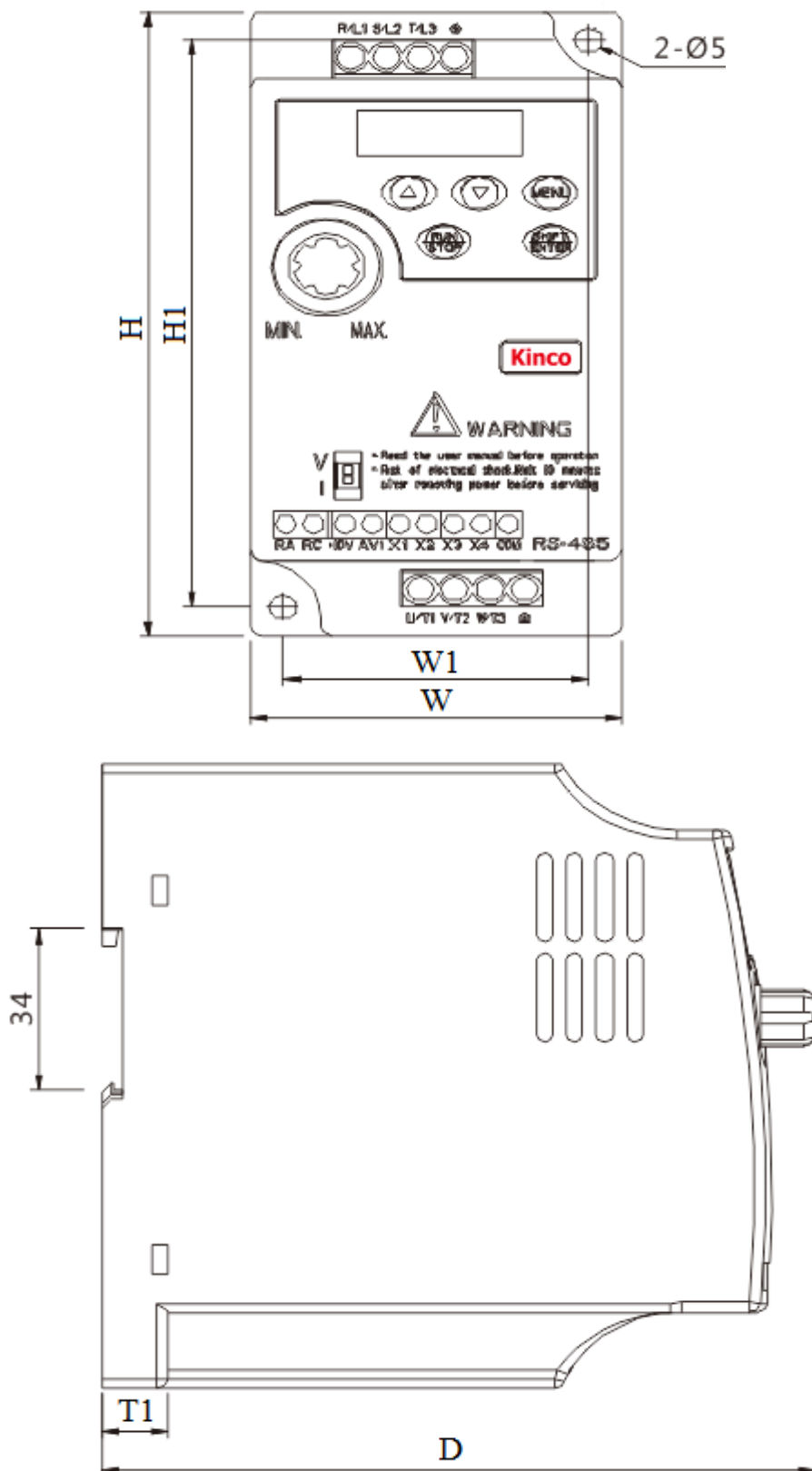
Рис. 2-2 CV20-2S-0004G ~ CV20-2S-0007G
