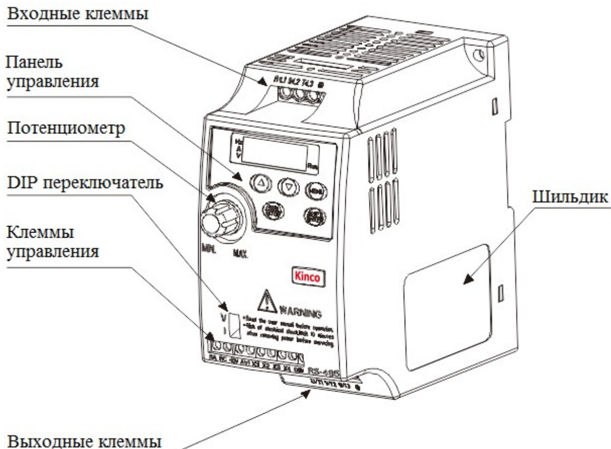
Рис. 2-1. Конструкция ЧРП
