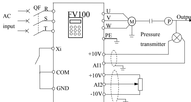
Рис. 6-38 Аналоговая система управления с обратной связью с внутренним замкнутым контуром
