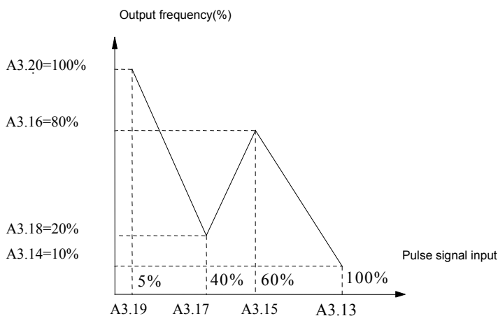
Рис. 6-10. Аналоговый сигнал, вход 1
