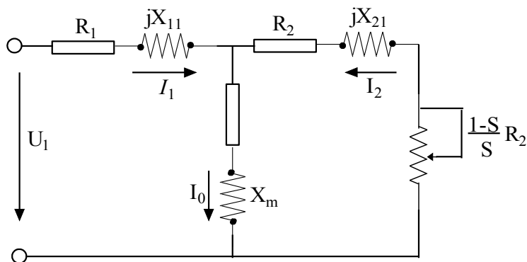
Рис. 6-33. Схема замещений двигателя
