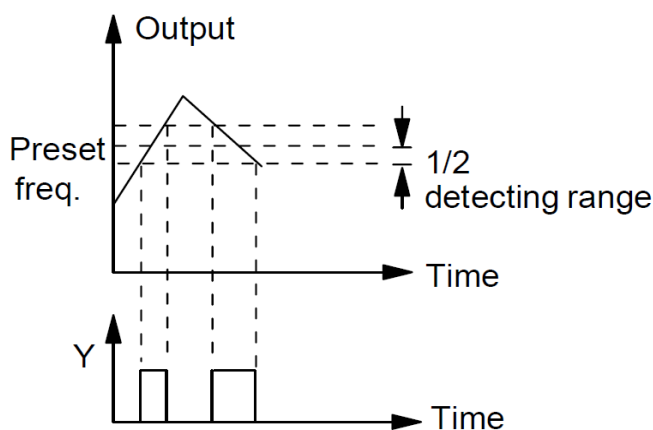
Рис. 6-26. Входной сигнал частоты
