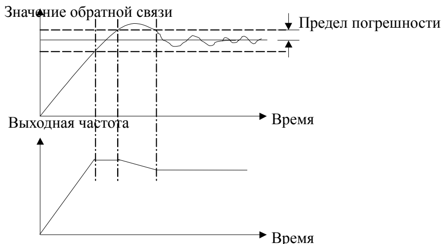
Рис. 6-42. Предельная погрешность
