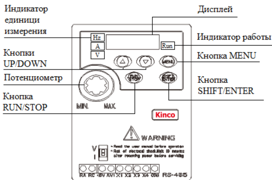
Рис. 5-1 Панель управления
