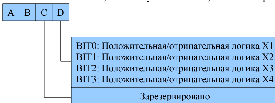
Рис. 6-24 Положительная и отрицательная логика клемм
