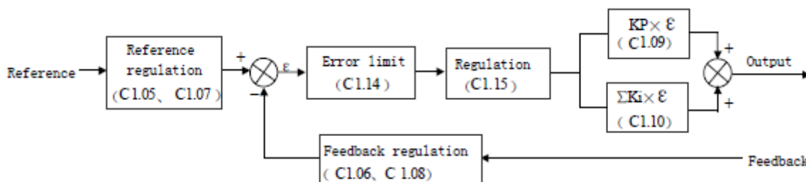
Рис. 6-39. Принципиальная схема процесса управления с обратной связью
