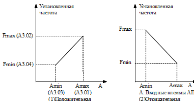
Рис. 6-8. Частота, соответствующая минимальной точке кривой
