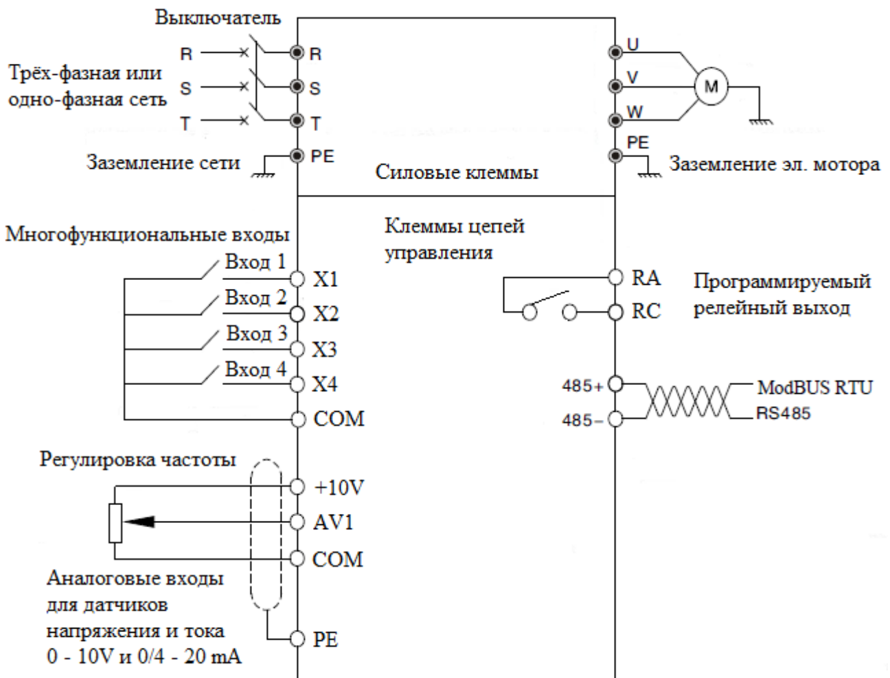
Рис. 4-1 Основная схема подключения
