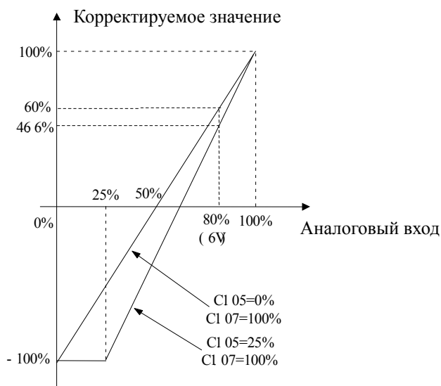
Рис. 6-41. Кривая управления относительным значением
