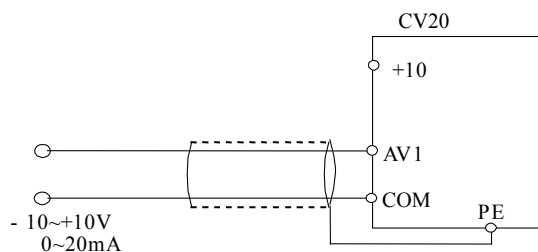
Рис. 4-3 Подключение клеммы AV1
