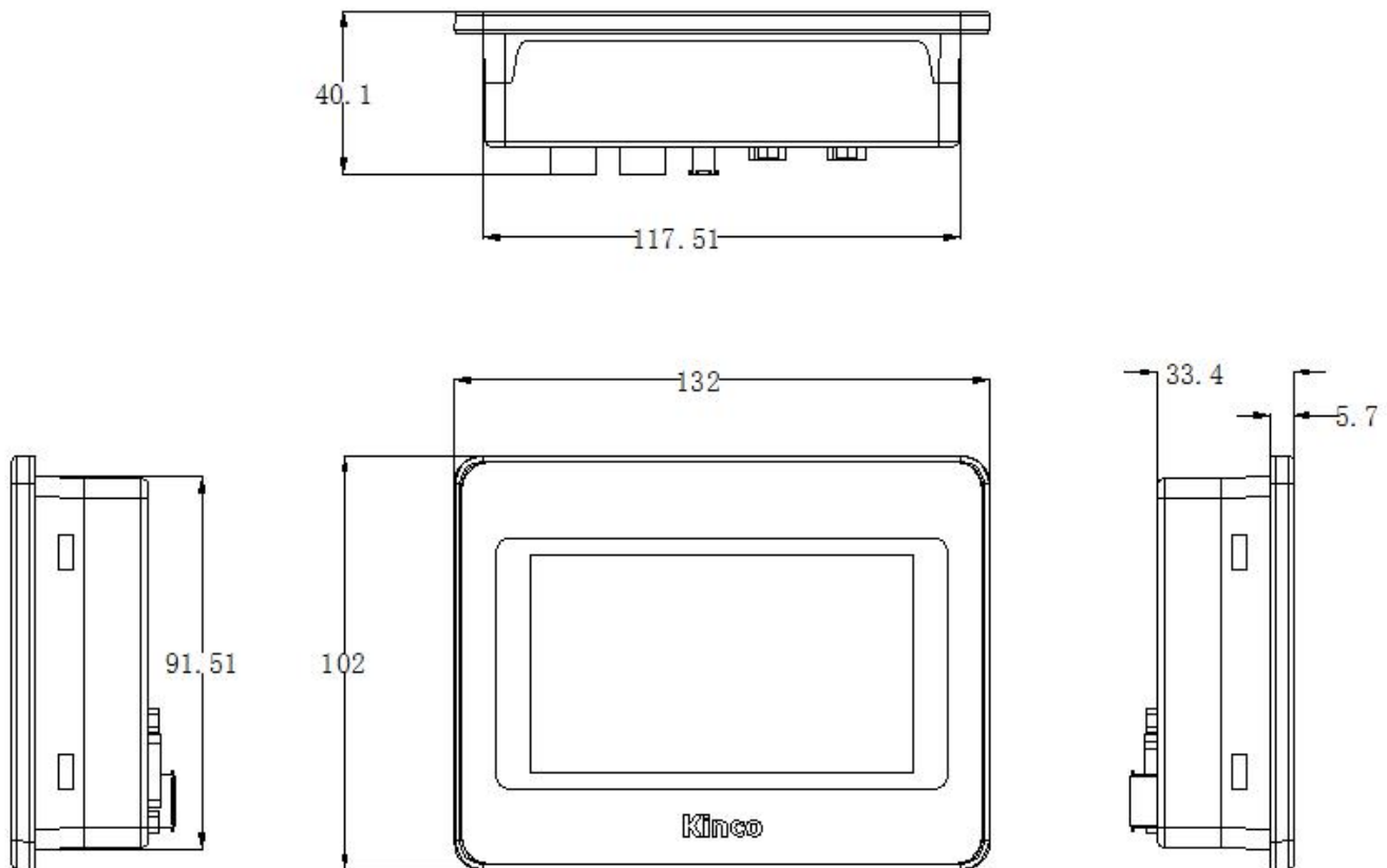
Рис. 2-7 Размеры HP043-20DT
