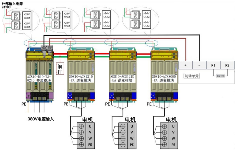
图 3-4 多机并联系统接线示意图
