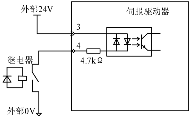
图 3-7 继电器输出的接线示例
