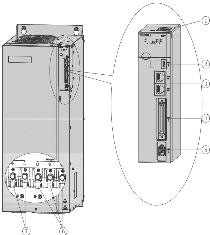
图 3-7（b） SD810 大功率逆变单元结构布局
