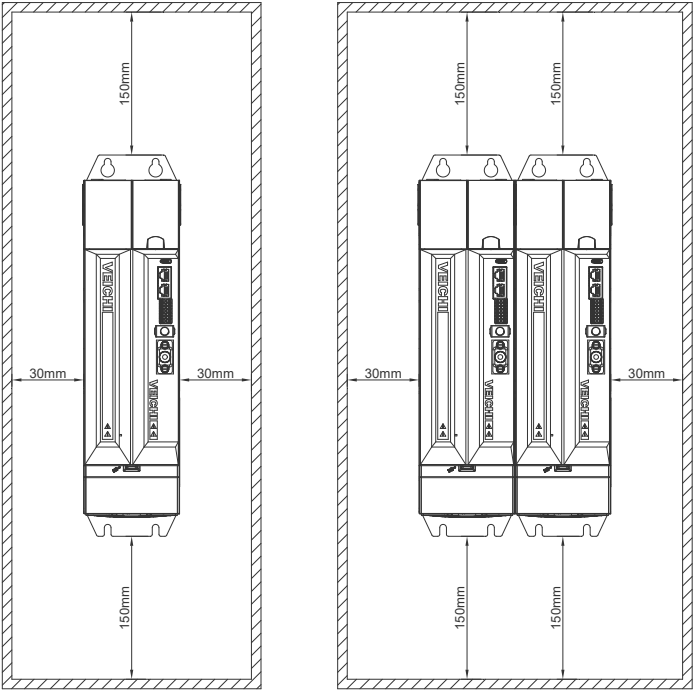
图 3-2(a) SD810 系列逆变单元安装示意图
