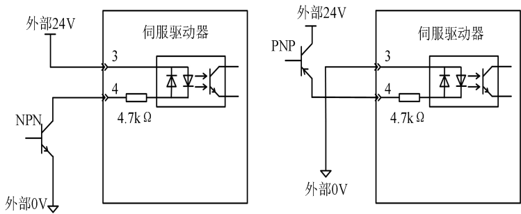
图 3-8 NPN/PNP 的集电极开路的连接示例
