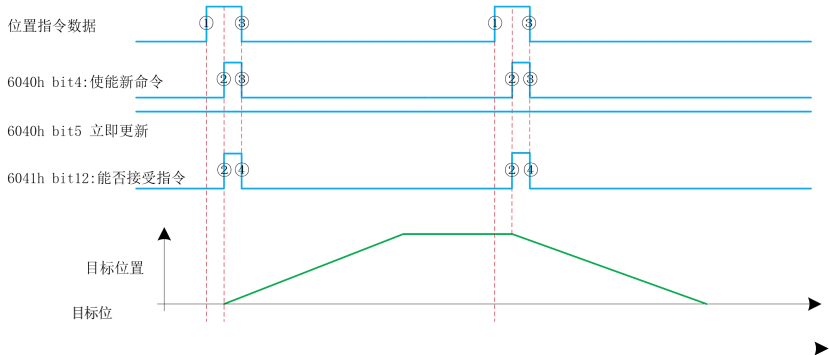
立即更新型时序图
