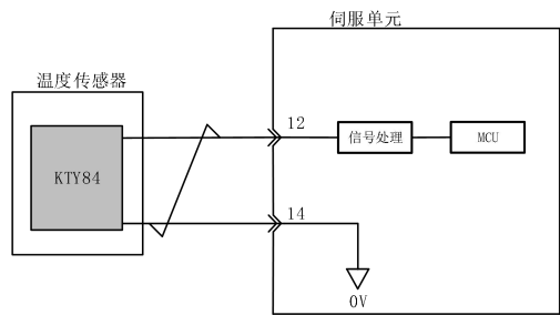
图 3-12 温度传感器连接示例
