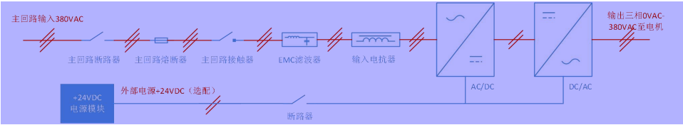
图 3-3 系统整体接线示意图
