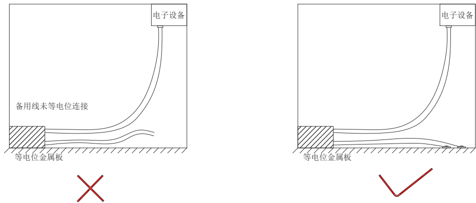
图 12-4 多芯电缆中有芯剩余时的处理方法示意图
