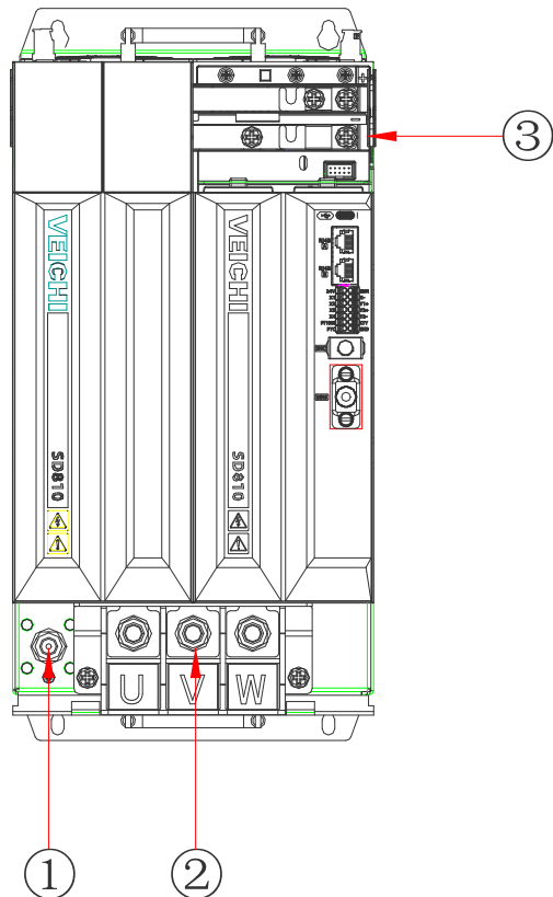
图 3-6 SD810 系列逆变单元主回路端子分布图
