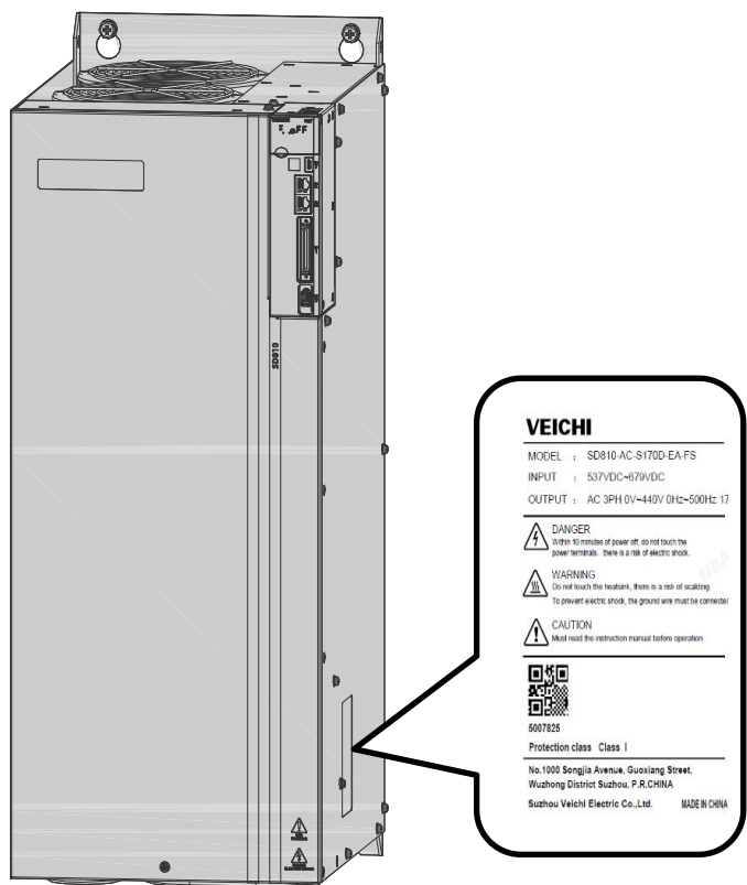
图 2-2 SD810 大功率结构逆变单元铭牌
