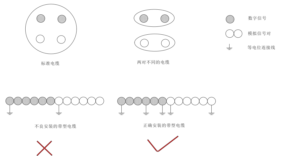
图 12-2 不同类型信号电缆分开排布示意图
