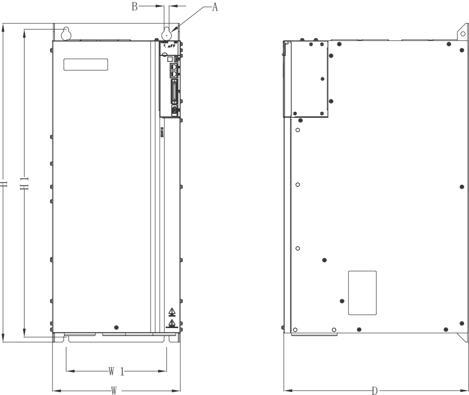
图 3-1(b) SD810 系列大功率逆变单元尺寸图
