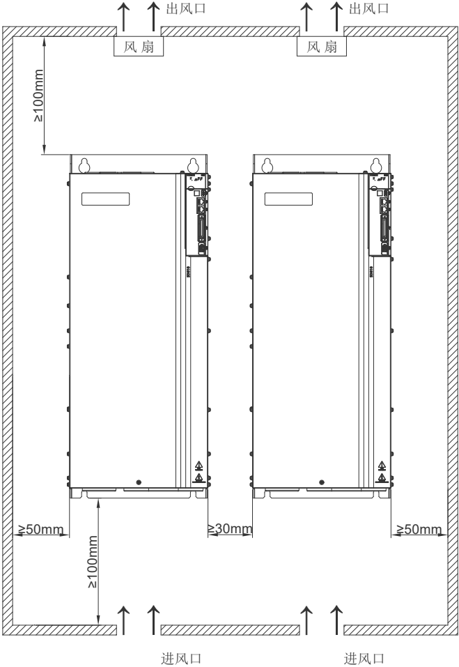
图 3-2 (b) SD810 系列大功率逆变单元安装示意图
