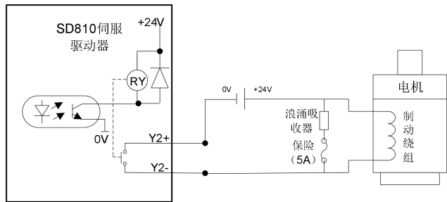
图 3-11 抱闸输出连接示例
