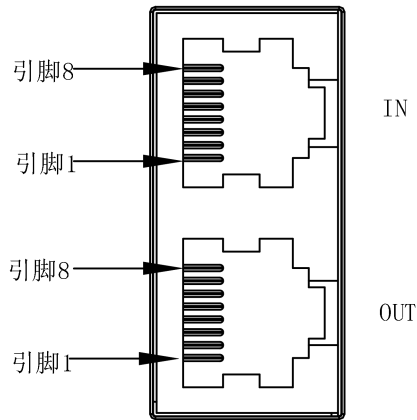
图 8.1 引脚定义 表 8-2 通信信号连接器引脚定义
