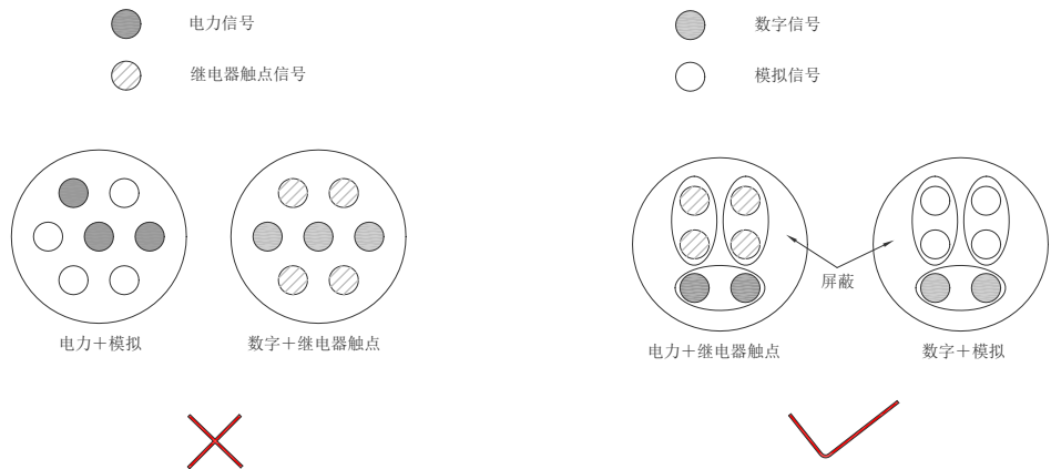
图 12-3 多芯电缆布线示意图
