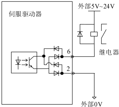
图 3-9 继电器输出的连接示例
