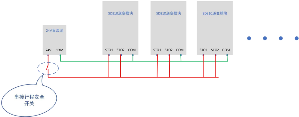
图 3-14 多台并机 STO 接线图
