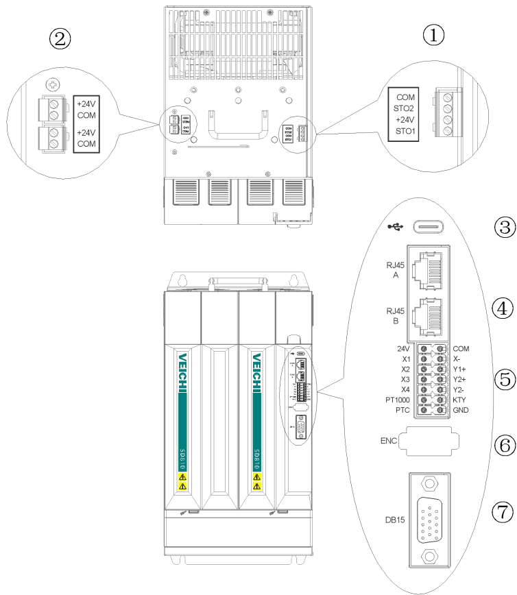
图 3-7（a） SD810 逆变单元结构布局 表 3-5（a） 系列逆变单元端子分布注释表 2
