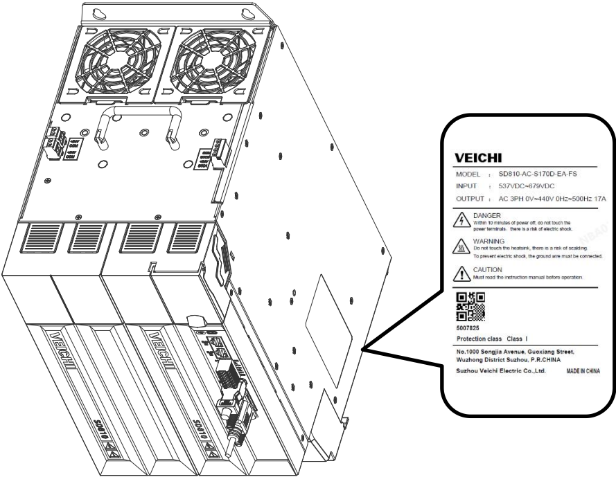
图 2-1 SD810 V3S 结构基本逆变单元铭牌
