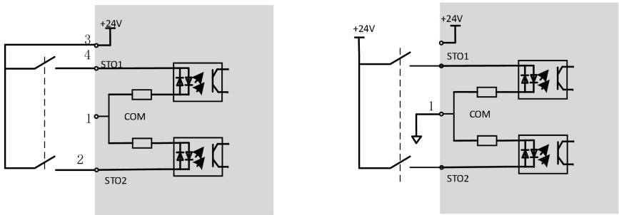
使用驱动器内部 24V 电源的接法
