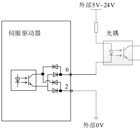
图 3-10 光耦输出的连接示例
