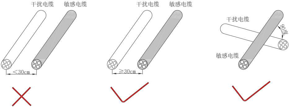
图 12-1 干扰电缆与敏感电缆电线布线示意图
