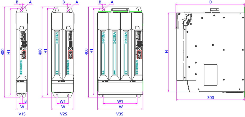
图 3-1(a) SD810 系列逆变单元尺寸图
