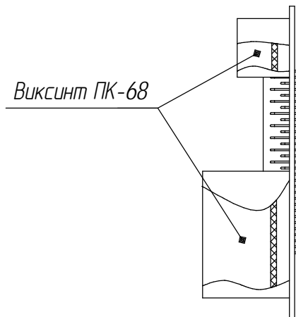
Устройство искробезопасного барьера ИБЯЛ.411613.036
