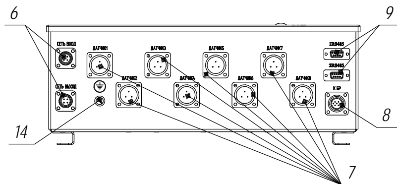
Вид снизу
